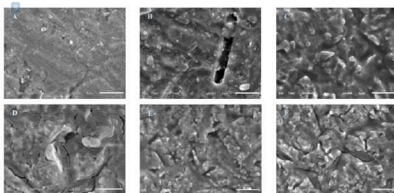
Gambar 6. Hasil uji SEM dengan perbesaran 5000x pada sampel: A) sebelum perlakuan; B) tanpa sandblasting ; C) sandblasting 500 kPa; D) sandblasting 600 kPa; E) sandblasting 700 kPa; dan F) sandblasting 800 kPa
