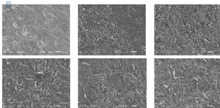
Gambar 5. Hasil uji SEM dengan perbesaran 1000x pada sampel: A) sebelum perlakuan; B) tanpa sandblasting ; C) sandblasting 500 kPa; D) sandblasting 600 kPa; E) sandblasting 700 kPa; dan F) sandblasting 800 kPa
