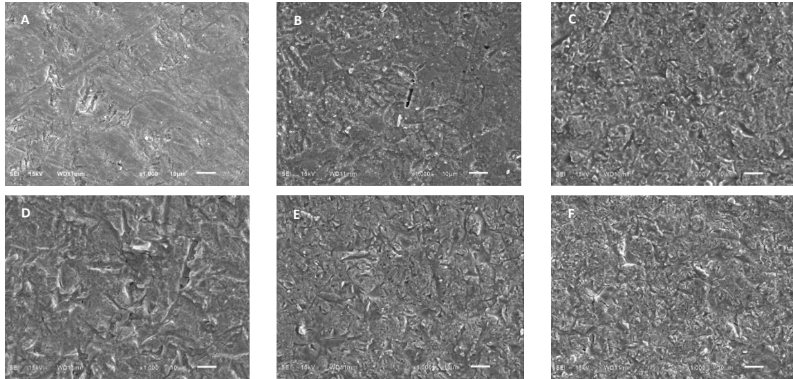
Gambar5. Hasil uji SEM dengan perbesaran 1000x pada sampel: A) sebelum perlakuan; B) tanpa sandblasting ; C) sandblasting 500 kPa; D) sandblasting 600 kPa; E) sandblasting 700 kPa; dan F) sandblasting 800 kPa
