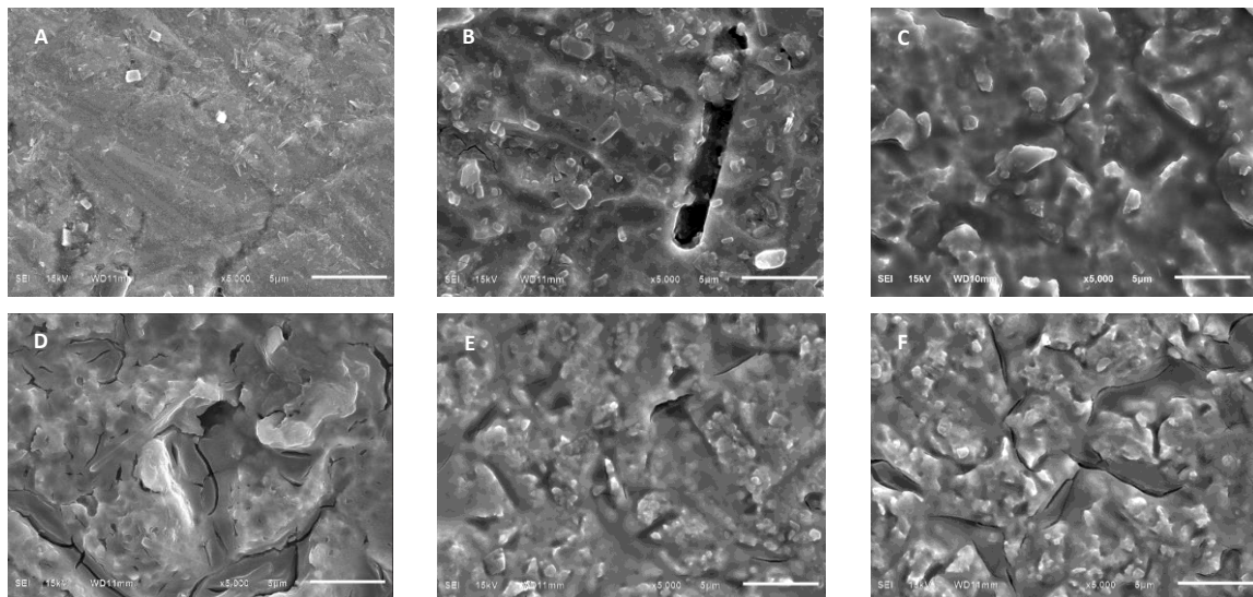
Gambar6. Hasil uji SEM dengan perbesaran 5000x pada sampel: A) sebelum perlakuan; B) tanpa sandblasting ; C) sandblasting 500 kPa; D) sandblasting 600 kPa; E) sandblasting 700 kPa; dan F) sandblasting 800 kPa
