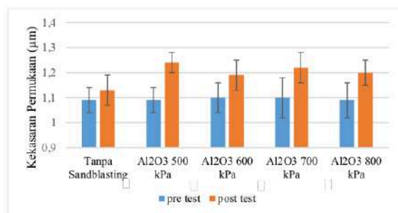
Gambar 2. Grafik nilai rerata kekasaran permukaan titanium alloy sebelum dan setelah perlakuan
