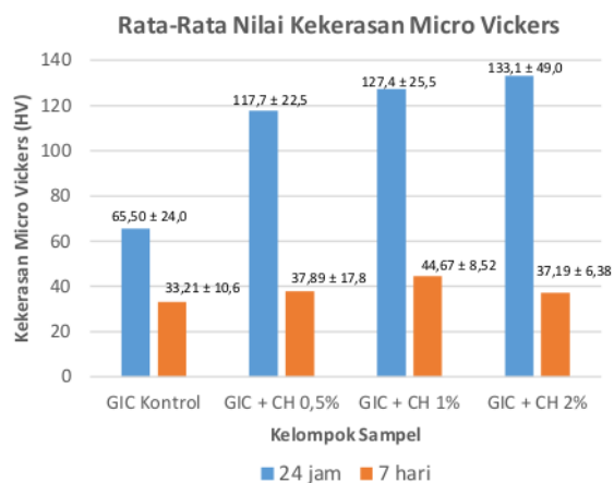
Gambar 3 Nilai kekerasan permukaan dari GIC Kontrol, GIC+NCH 0,5wt%, GIC+NCH 1wt%, GIC+NCH 2wt% dengan waktu perendaman 24 jam dan 7 hari ( p < 0,05 ; n = 10 )
