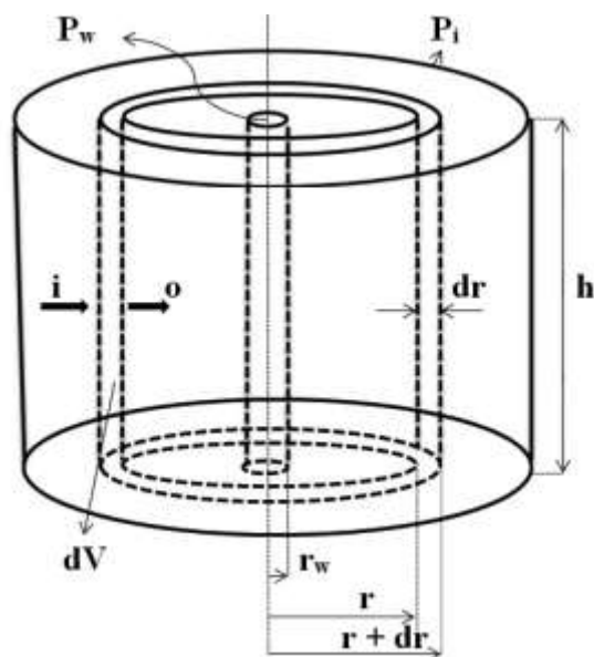
Gambar 1. Aliran radial
