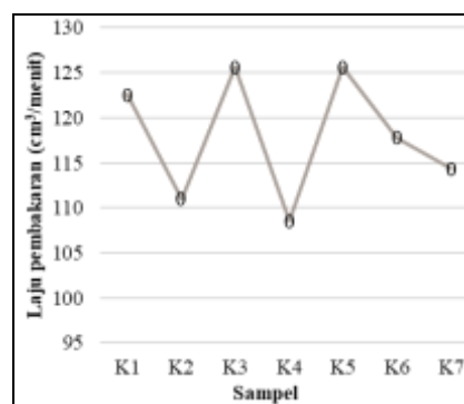
Gambar 4. Laju pembakaran briket
