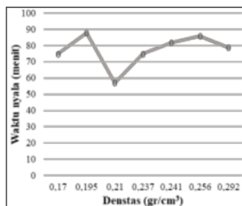
Gambar 3. Grafik waktu nyala briket berdasarkan nilai densitasnya
