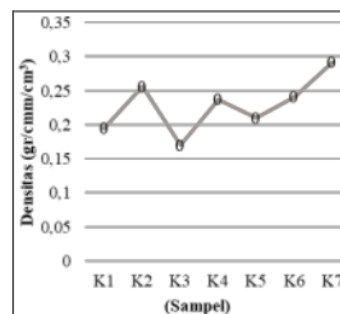
Gambar 2. Grafik densitas briket berdasarkan komposisi penyusunnya
