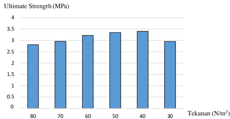
Gambar 4. Pengaruh Tekanan terhadap Ultimate Strength
