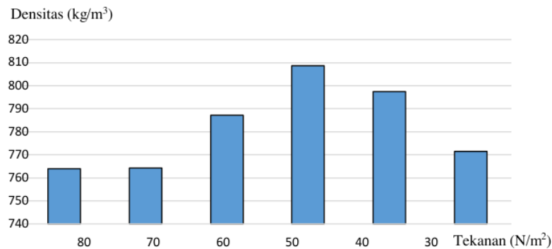
Gambar 2. Pengaruh Tekanan terhadap Densitas
