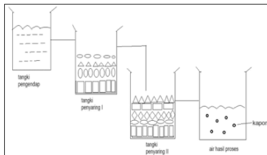
Gambar 6. Bagan Teknik Pengelolaan Air
