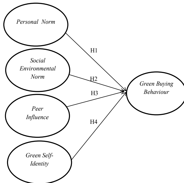
Gambar 1. Rerangka Pemikiran
