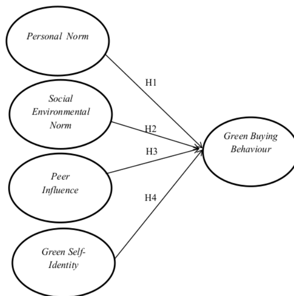
Gambar 1. Rerangka Pemikiran
